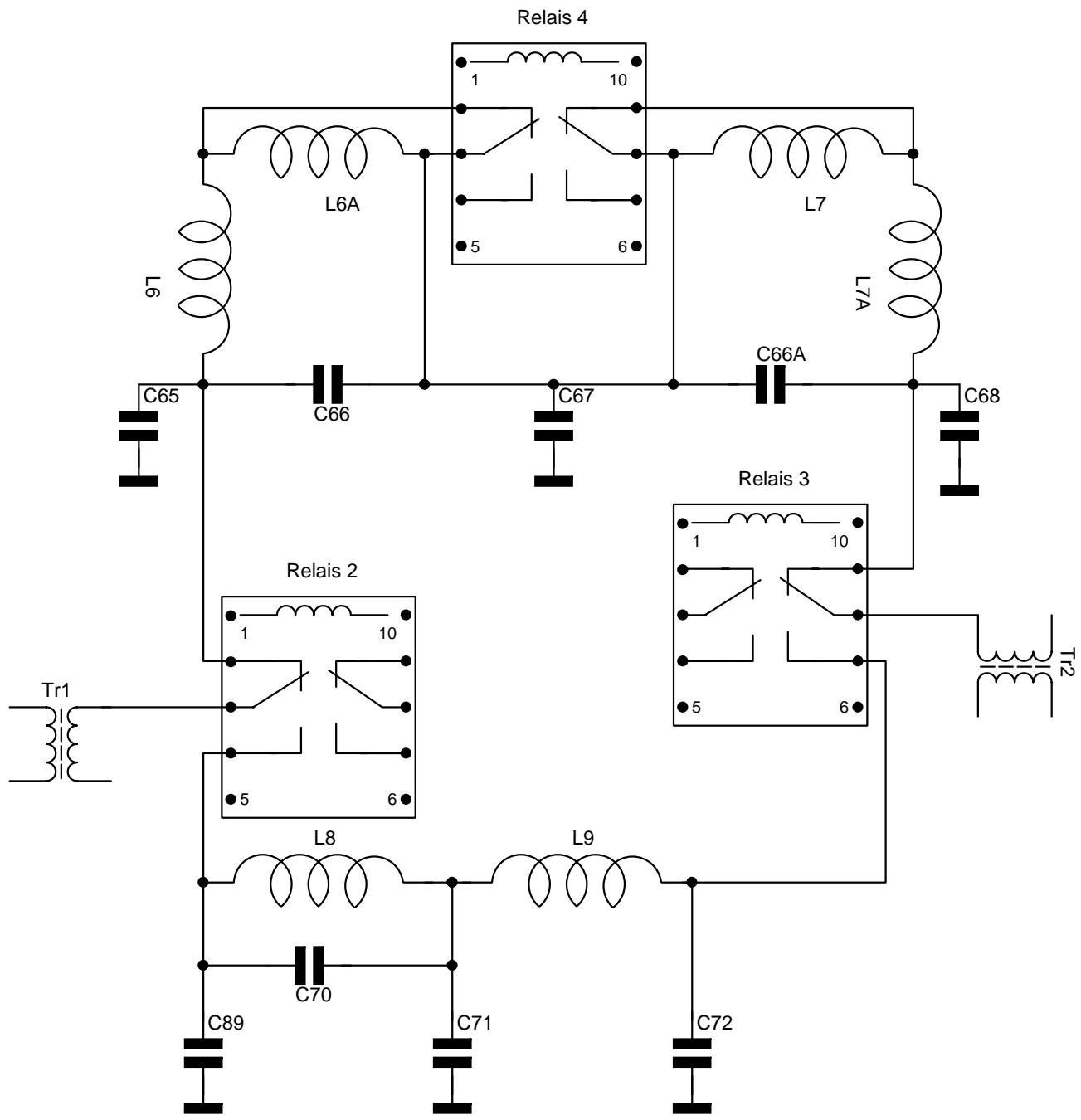
BCR Tiefpasserweiterung Prototyp 23.3.06
